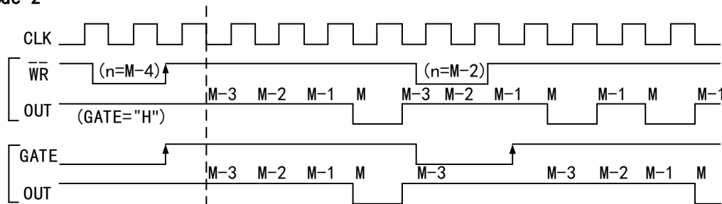
图7-4-3 计数方式2时序图
