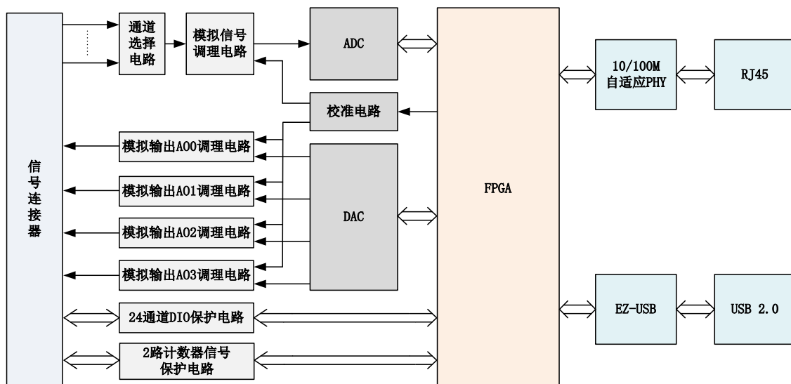
图 2-2-1 USB563X 系统框图
