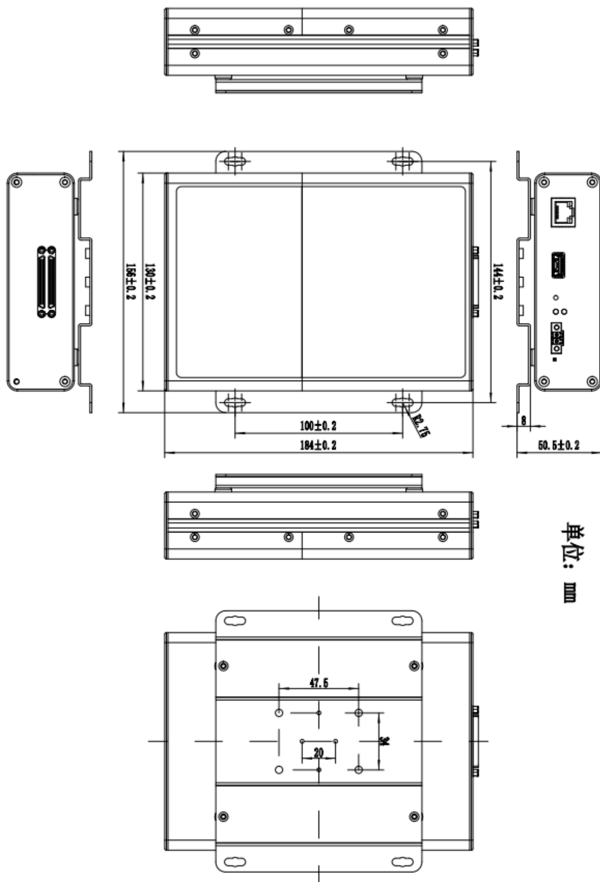
图 3-2-2 USB563X-V 外壳尺寸图
