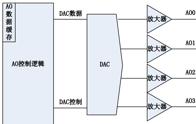
图 5-1-1 AO 功能框图
