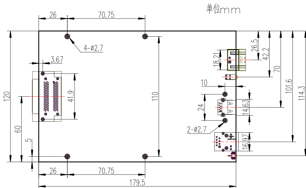
图 3-2-3 USB563X-V 内部尺寸图
