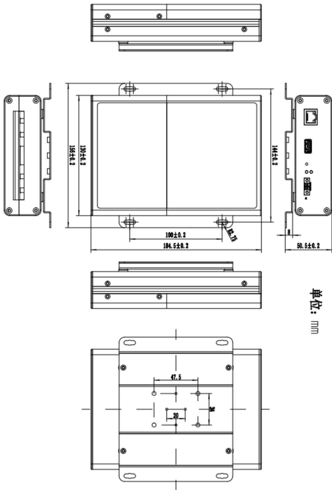
图 3-2-1 USB563X-D 外壳尺寸图
