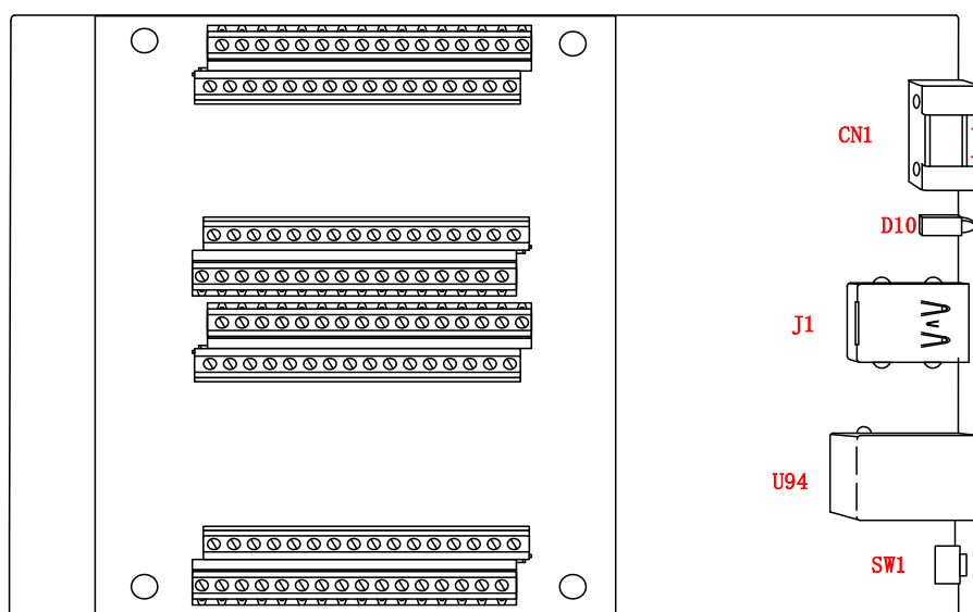
图 3-2-4 USB563X-D 内部示意图
