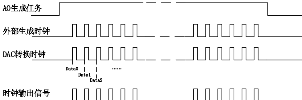
图 5-6-3 外时钟时序图
