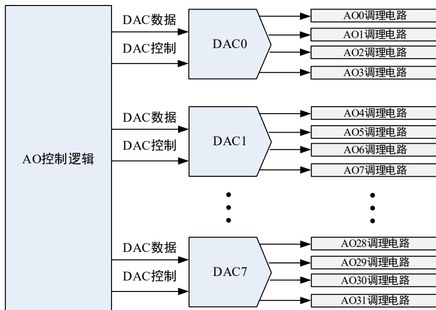
图 5-1-1 AO 功能框图
