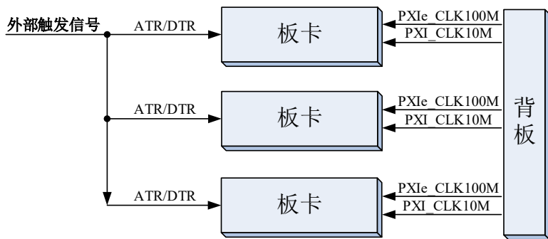
图 4-10-1 主从卡级联
