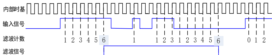
图 6-9-1 数字滤波
