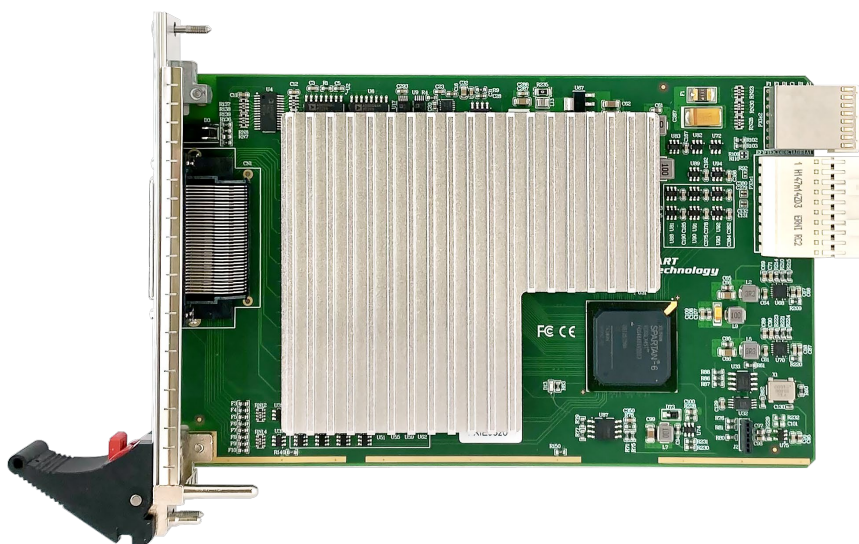
图 3-1-2 PXIe9320 正面图
