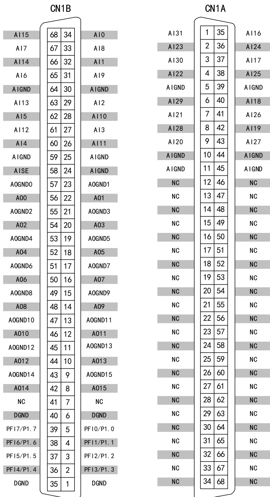
图 3-3-4 9321 连接器引脚定义
