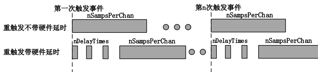
图 8-2-5 重触发
