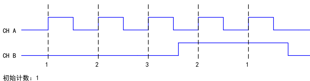
图 6-7-5 单脉冲编码
