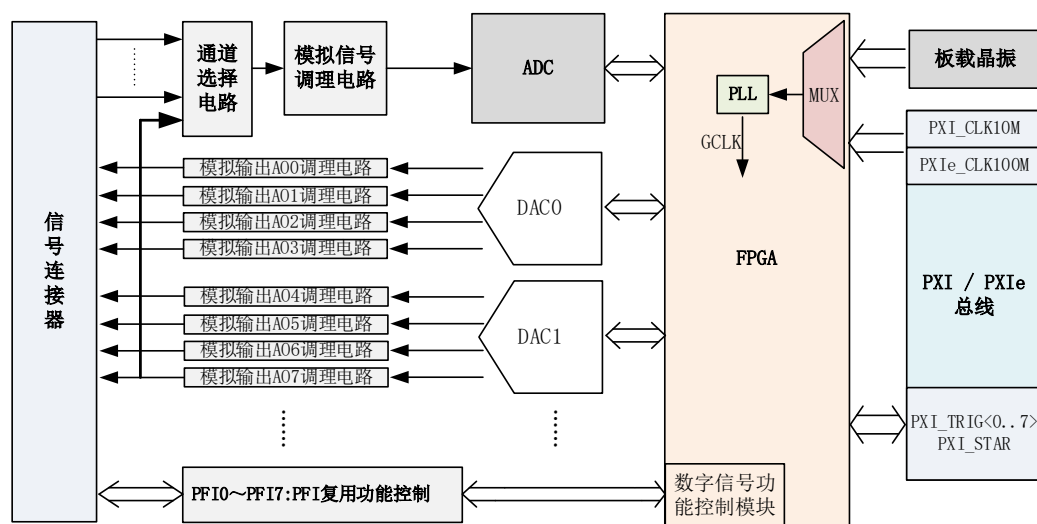
图2-2-1 932X系统框图
