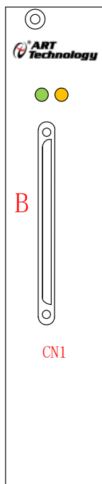
图 3-3-2 9322 单 VHDCI-68 连接器挡片示意图
