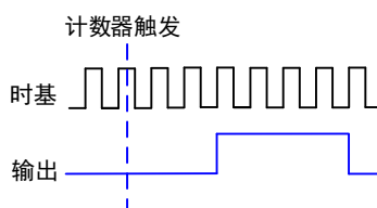
图 6-8-1 单脉冲生成
