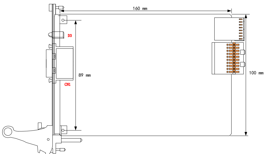
图 3-2-2 PXIe932X 板卡尺寸图
