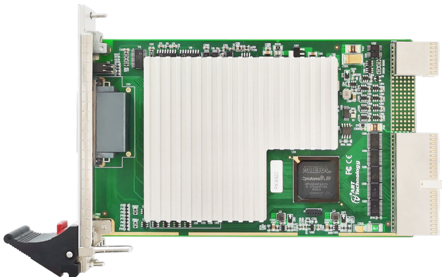
图 3-1-1 PXI9320 正面图
