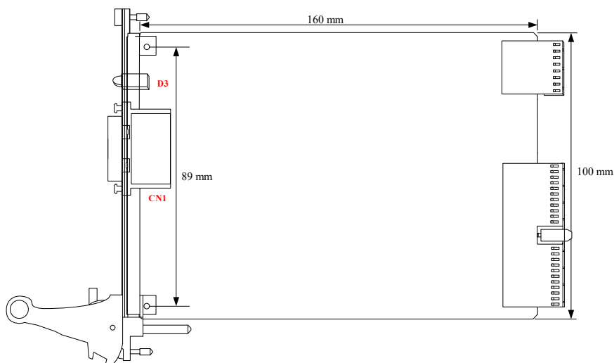
图 3-2-1 PXI932X 板卡尺寸图
