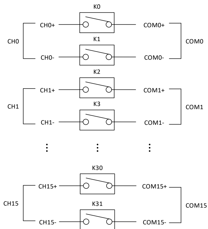
图 3-3-2 16-DPST 拓扑结构图
