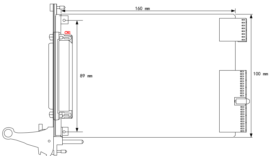
图 3-1-2 PXI2613 尺寸图
