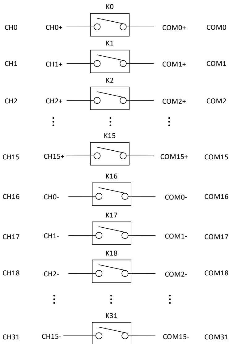
图 2-2-1 硬件框图
