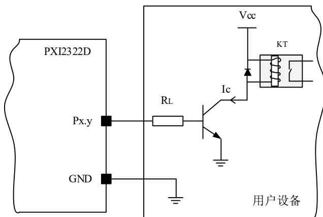
图 4-4-3 Sink 方式连线示意图, > 24mA
