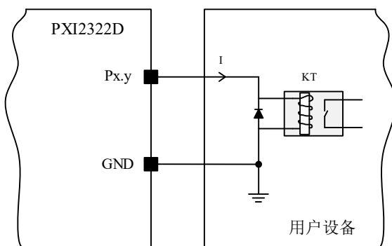
图 4-4-2 Source 方式连线示意图, < 24mA
