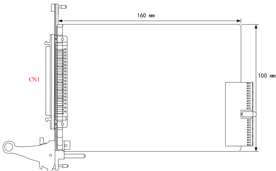
图 3-2-1 PXI2322D 尺寸图
