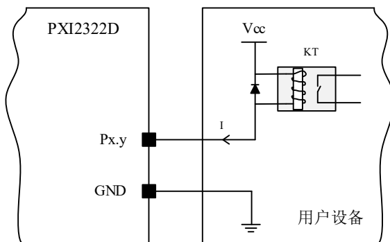
图 4-4-1 Sink 方式连线示意图, < 24mA
