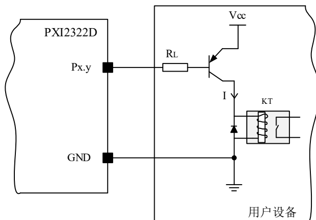
图 4-4-4 Source 方式连线示意图, > 24mA
