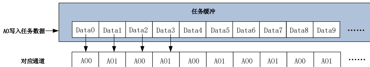
图5-5-2 AO多通道存储顺序
