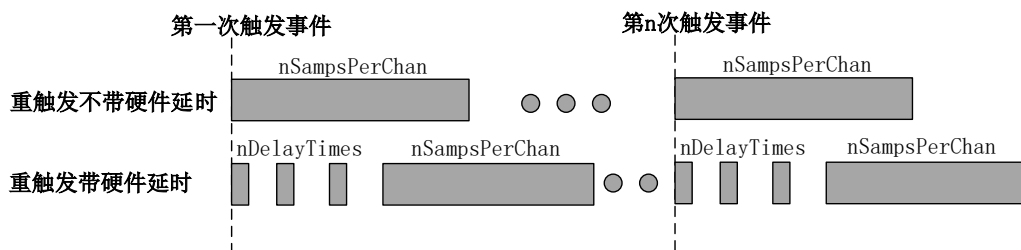
图 8-2-4 重触发
