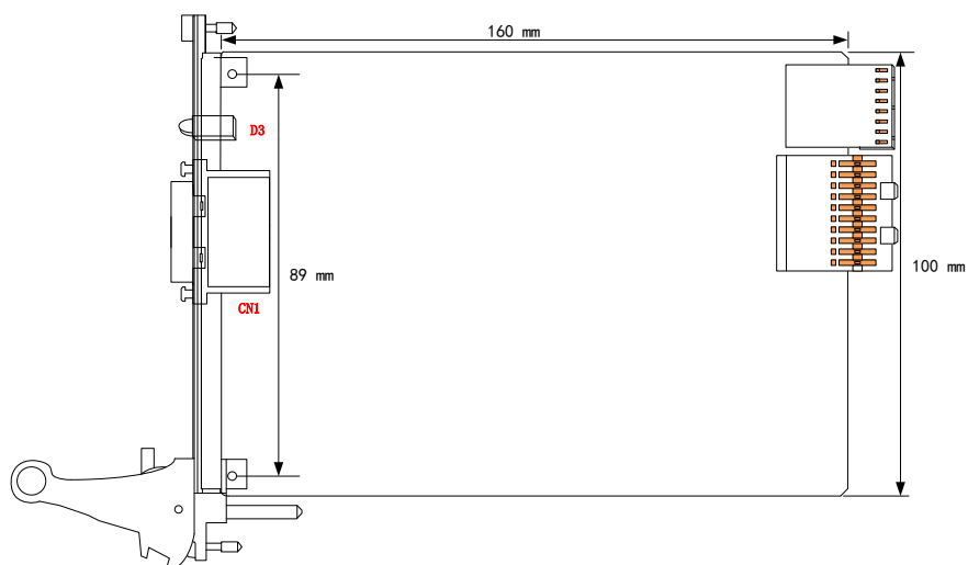
图 3-2-4 PXIe9774 板卡尺寸图
