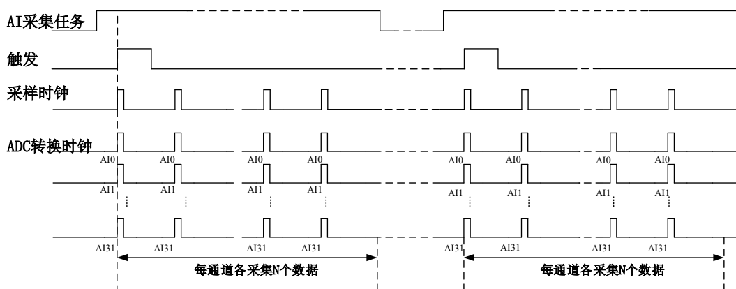
图 4-7-2 有限点采样
