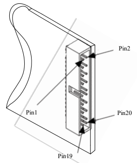
图 3-3-3 RTSI 的 Pinout 图
