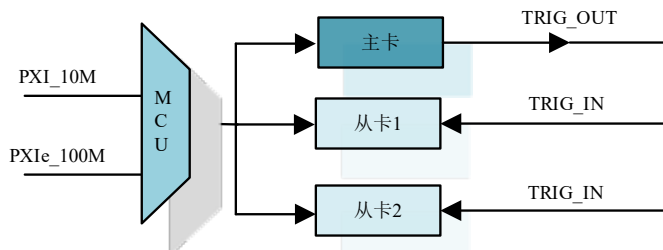
图 4-10-1 采用机箱背板的 PXI_10M 或 PXIe_100M 时钟信号作为时钟参考源
