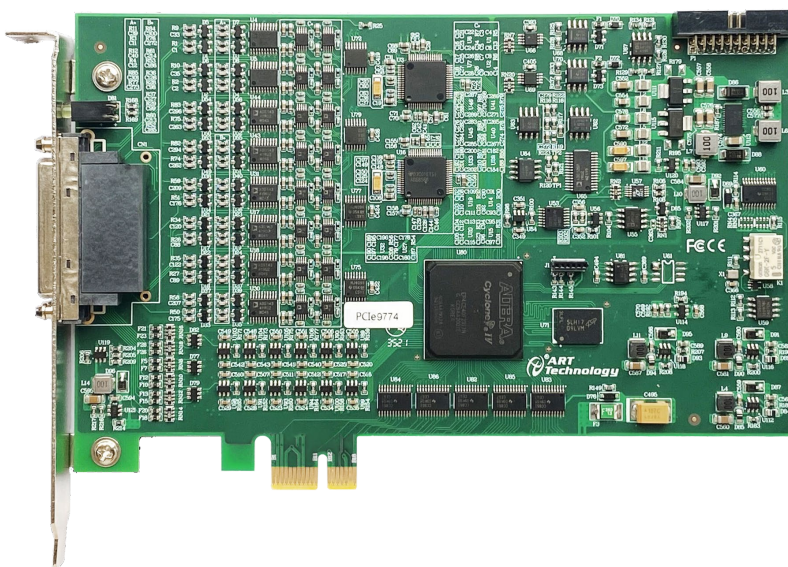
图 3-1-2 PCIe9774 外观图
