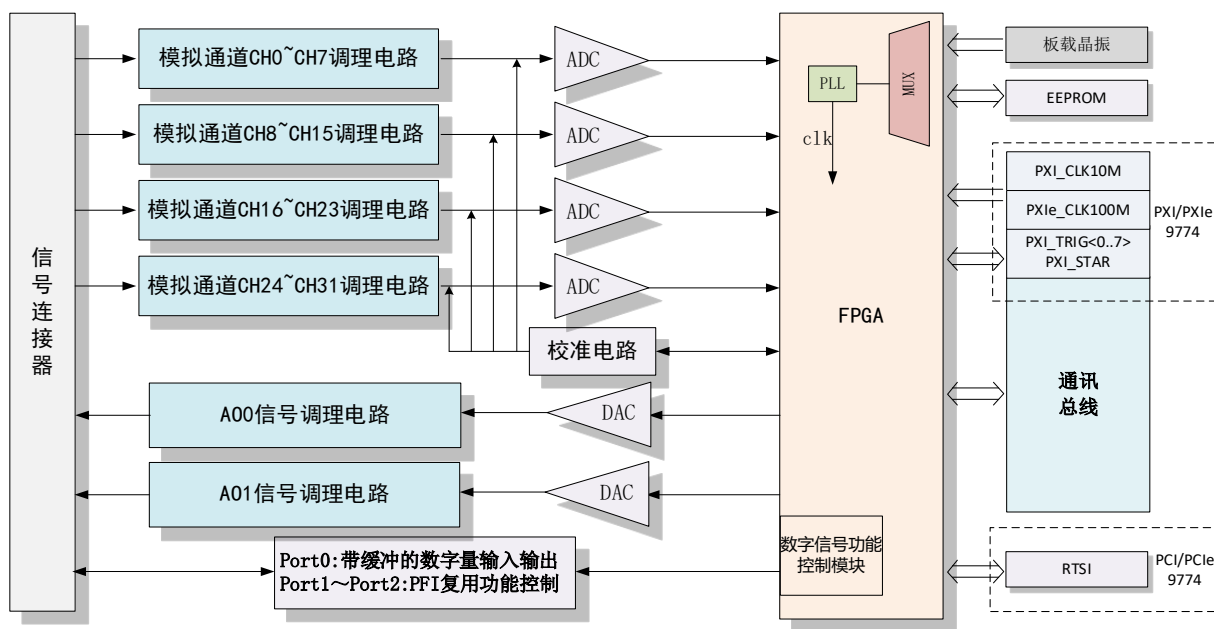
图2-2-1 9774板卡系统框图
