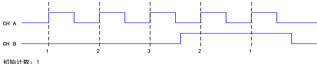
图 5-7-5 单脉冲编码
