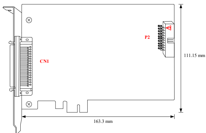
图 3-2-2 PCIe2880/A/B 板卡尺寸图
