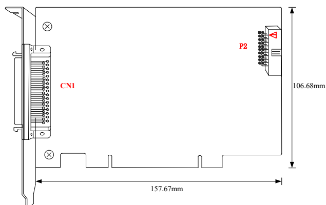
图 3-2-1 PCI2880/A/B 板卡尺寸图
