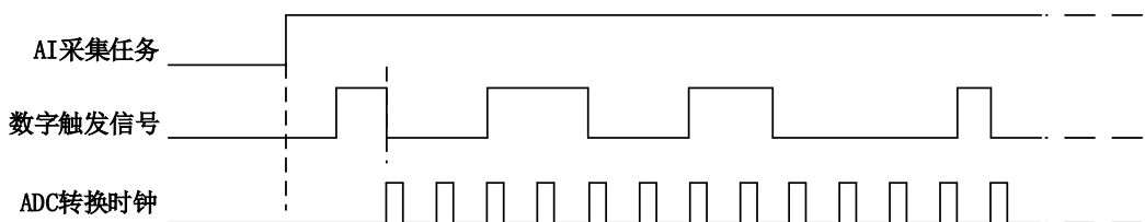
图 7-2-2 数字触发--下降沿触发
