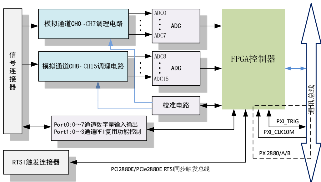
图2-2-1 2880/A/B 系统框图
