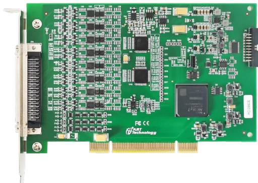
图 3-1-1 PCI2880/A/B 板卡外形图
