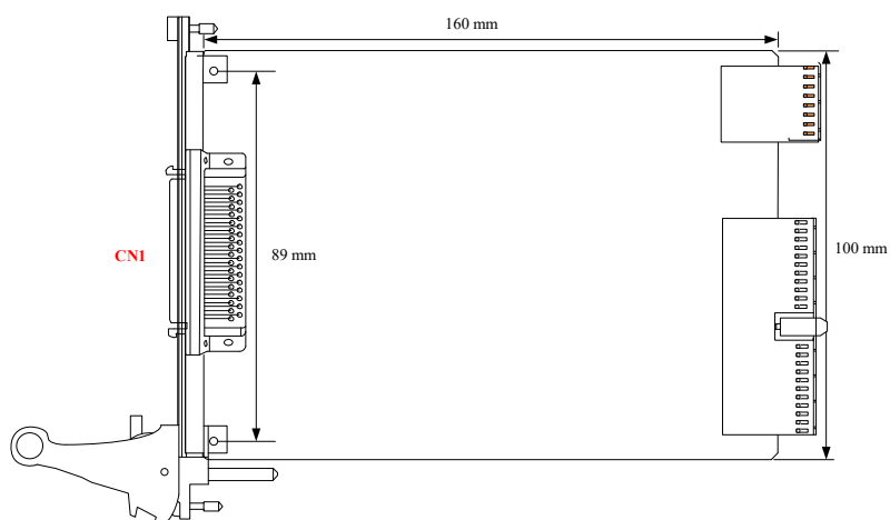
图 3-2-3 PXI2880/A/B 板卡尺寸图
