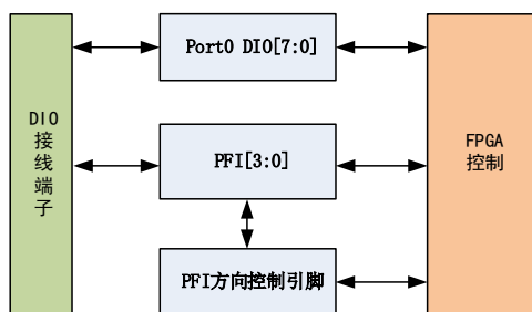
图6-1-1 DIO功能框图
