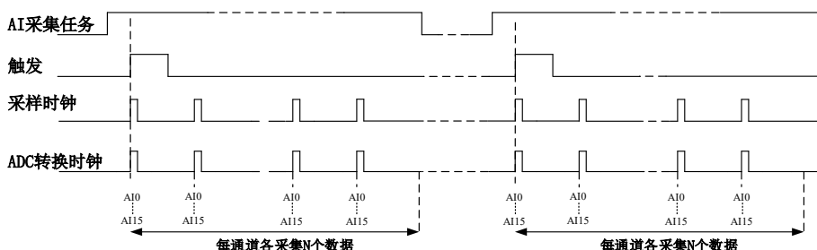
图 4-7-2 有限点采样
