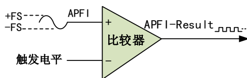
图7-3-4 模拟触发比较器
