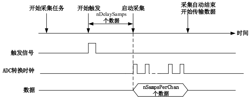
图 7-2-4 硬件延时触发
