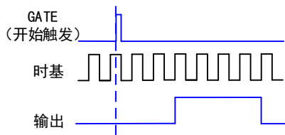
图 5-8-2 具有启动触发的单脉冲生成
