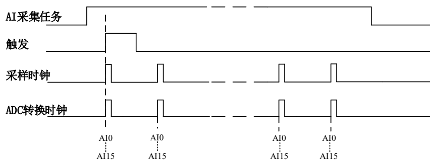
图4-7-3 时钟连续采样
