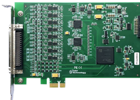
图 3-1-2 PCIe2880/A/B 板卡外形图
