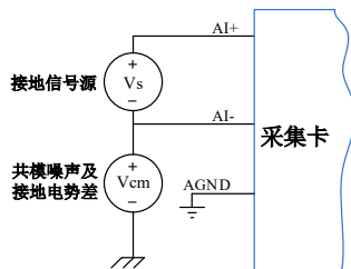
图 4-5-6 接地信号源的差分（DIFF）连接
