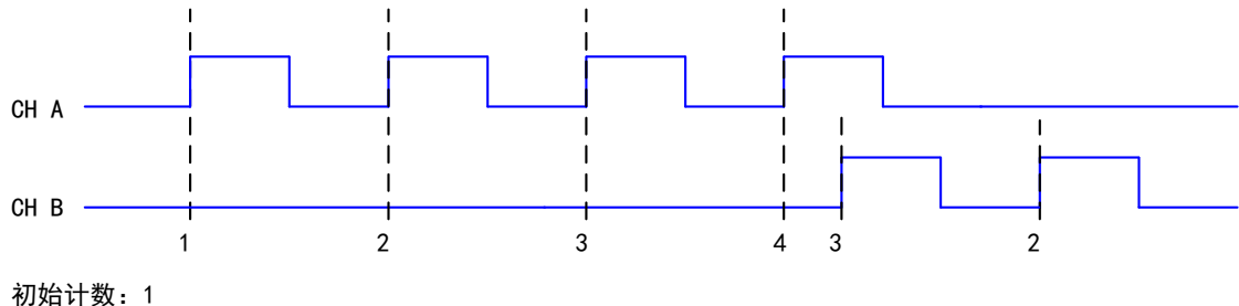
图 5-7-4 双脉冲编码
