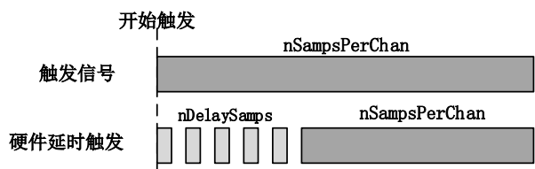
图 7-2-3 AI 硬件延时触发
