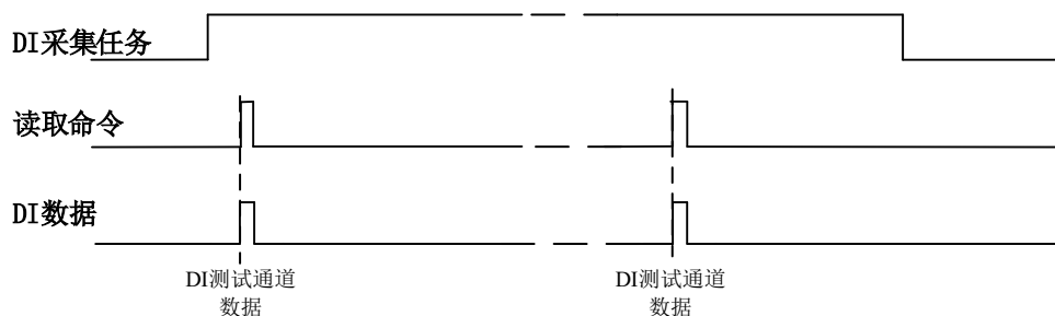
图6-5-1 按需单点采集
