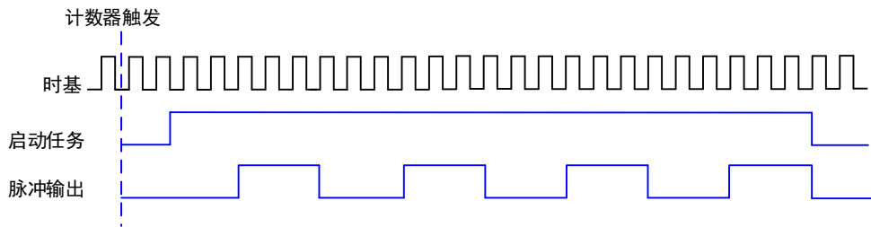
图 5-8-3 有限脉冲序列生成
