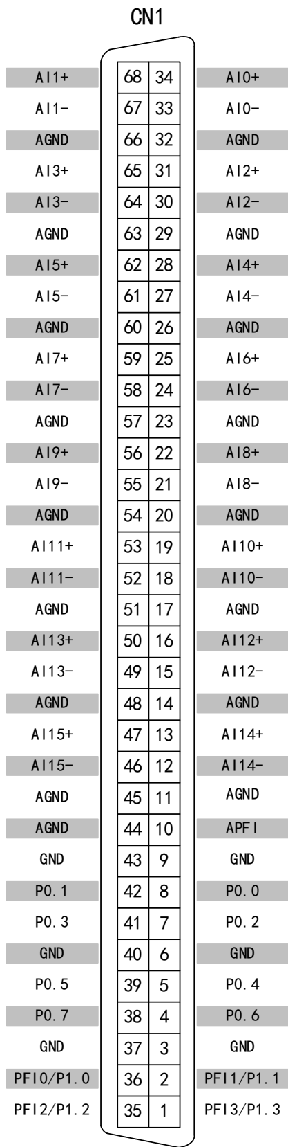
图 3-3-1 2880/A/B 管脚定义图
