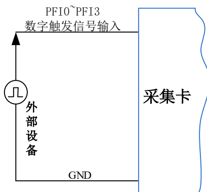
图7-3-6 数字触发连接方法
