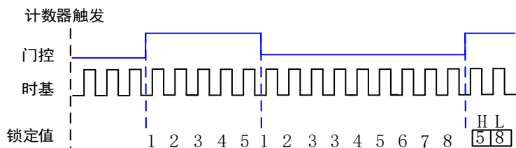
图 5-4-1 单（按需）脉冲测量
